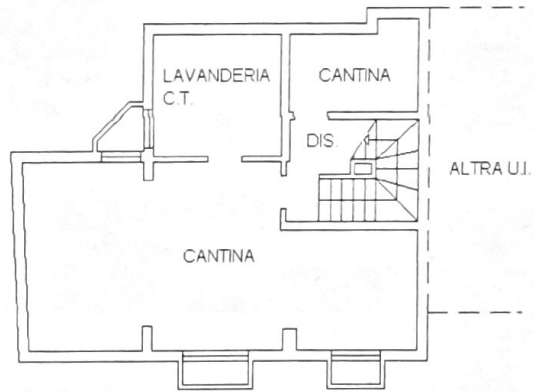
PIANTA PIANO INTERRATO H=230
